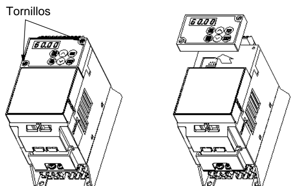
Figura 1-3-4 Retiro del teclado
