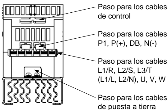
Fig 1-2-3a Vista de los terminales (hasta 4.0kW)
