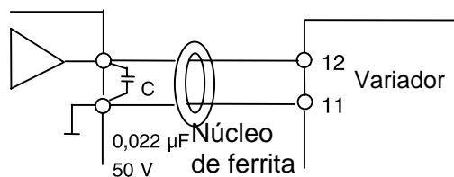
Figura 2-3-4 Ejemplo de prevención de ruidos
