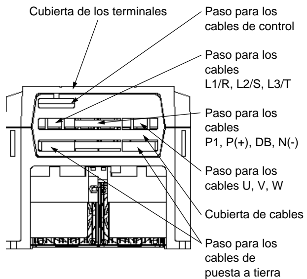
Fig 1-2-4 Vista de los terminales (5.5, 7.5kW)
