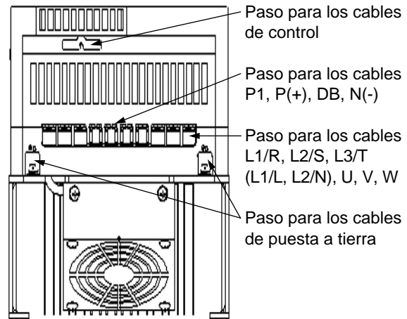
Fig 1-2-3b Vista de los terminales (bis 4.0kW)
