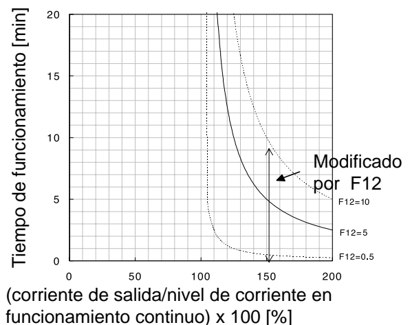
Característica típica corriente – tiempo de reacción
