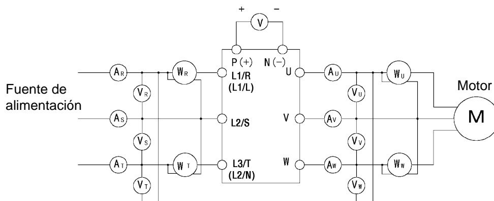
Figura 8-3-1 Conexión de los medidores
