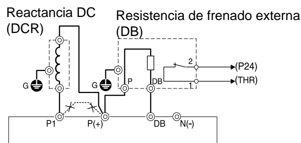
Figura 2-3-2 Conexión
