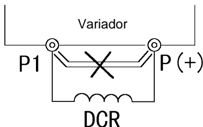
Figura 2-3-1 Conexión de una reactancia DC
